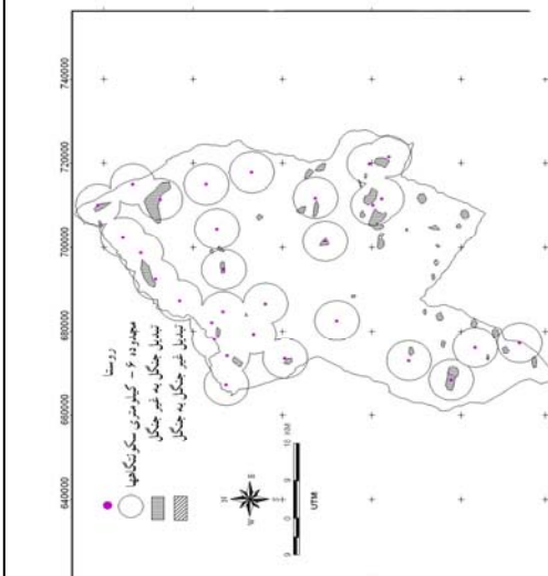
شکل ۸ - نقش عوامل سکو تنگناهی در روند تغییر جنگلهای ارسنجان مابین سالهای ۲۰۰۲-۱۹۸۷
