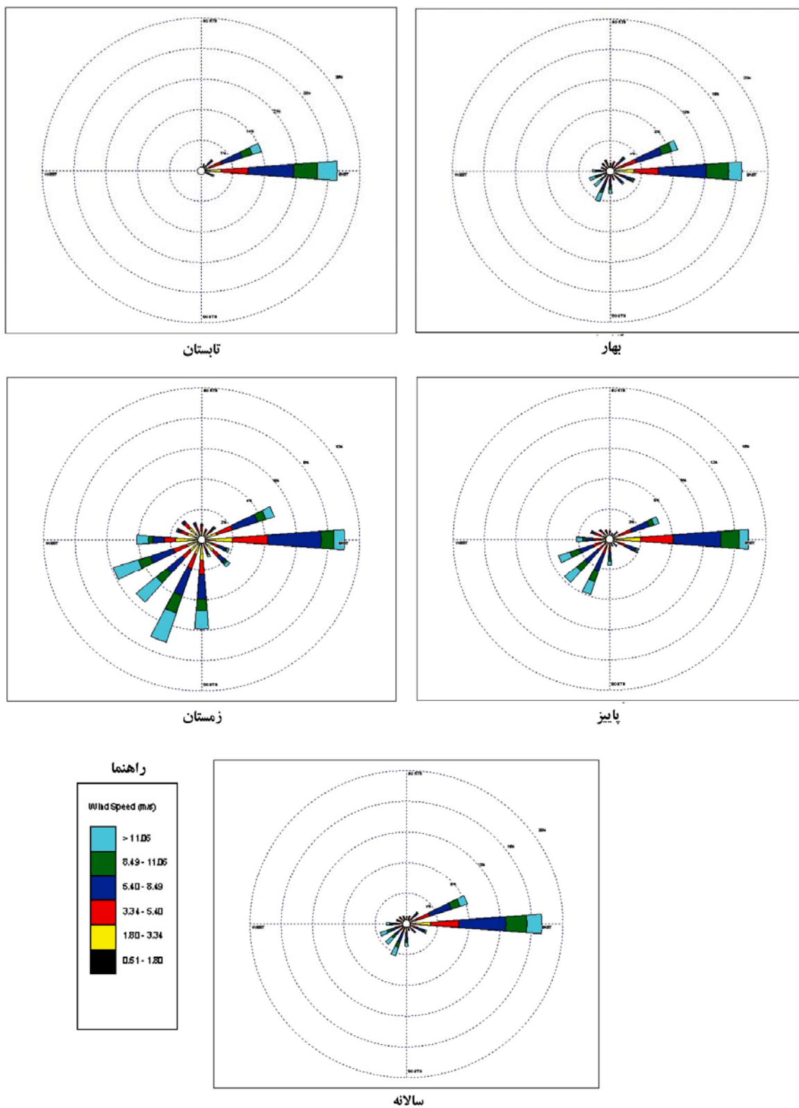
نمودار شماره ۱. گلباد فصلی و سالانه ایستگاه سینوپتیک اردبیل در دوره آماری ۱۹۹۰-۱۹۹۹
