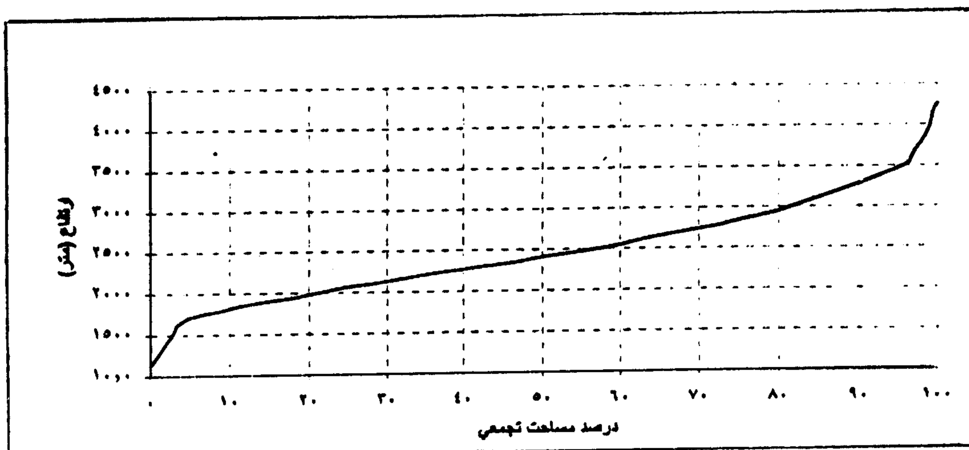
شکل ۱- منحنی تغییرات سطح با ارتفاع در حوضه آبریز طالقان (منحنی هیپسومتریک)
