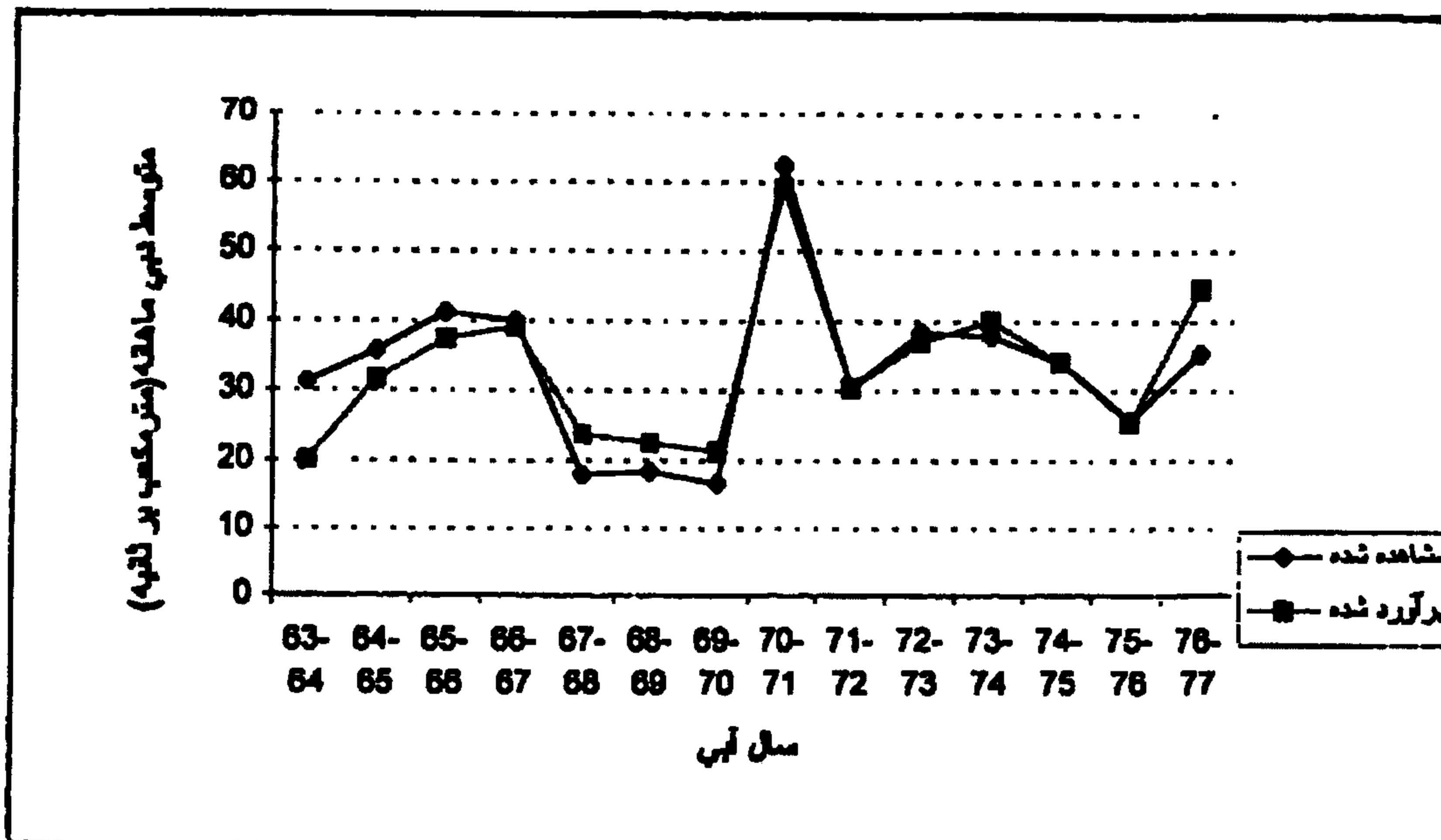
شکل ۳- مقایسه مقادیر دبی محاسبه شده با مقادیر مشاهده شده در خرداد ماه
