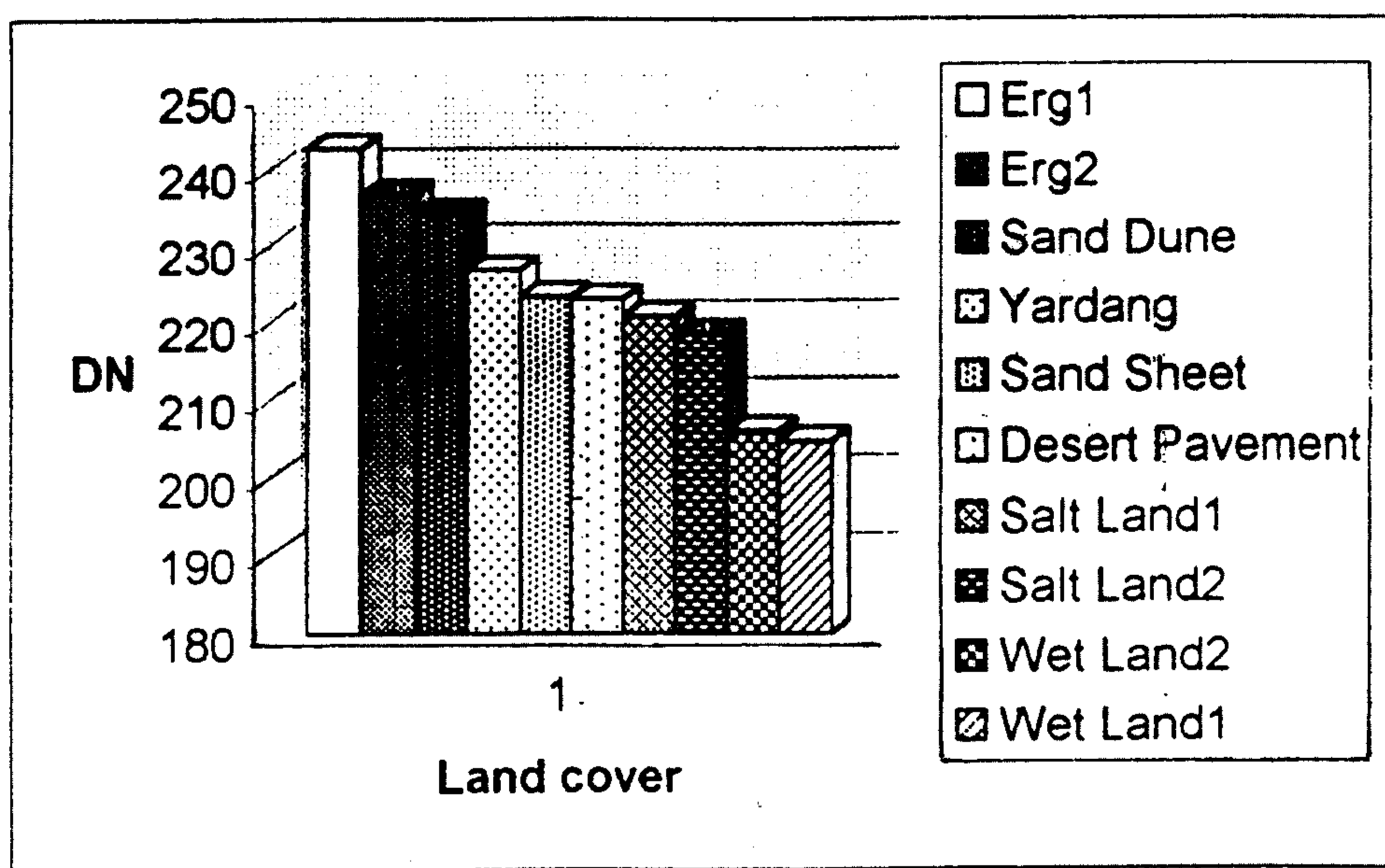
تصویر ۴- میانگین DN باند حرارتی (TM6) کلاس‌های آموزشی منطقه
