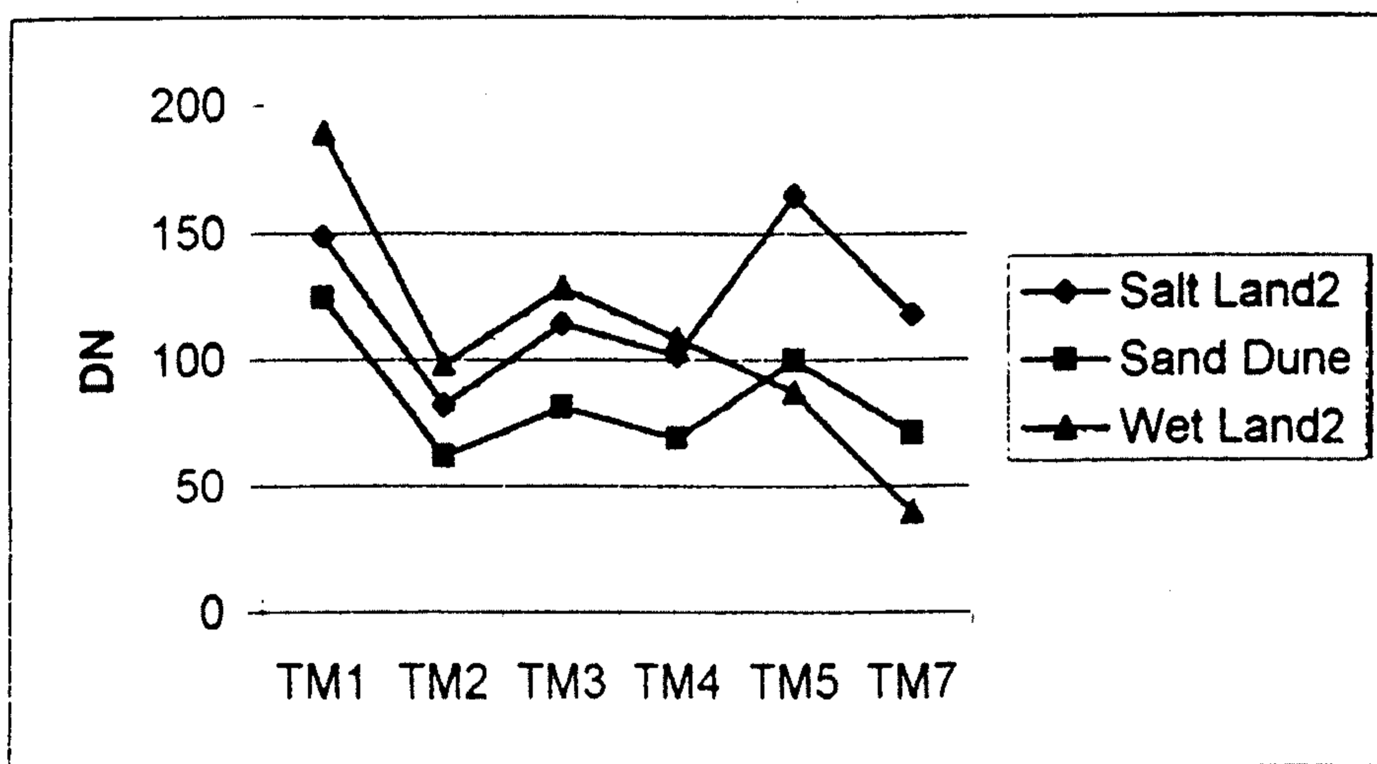
تصویر ۳- میانگین بازتاب‌های طیفی چند کلاس آموزشی
